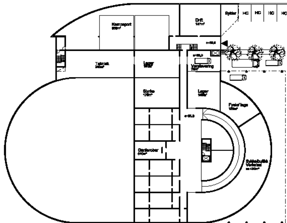
Skisse Velodrom 16.01.2017 - Plan 1 etg - NSW Sivilarkitekter MNAL
